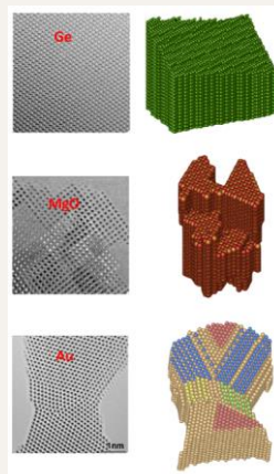
左排是奈米鎢晶、氧化鎂奈米顆粒及金奈米橋的 2D 原子影像，右排各為以上奈米顆粒重構的 3D 原子的斷層結構。
