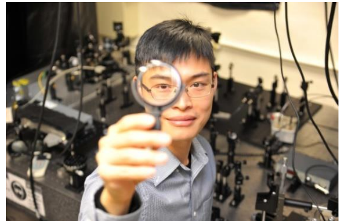
本校光電所劉昌樺老師研發出世界上最薄的介電質超平面透鏡
