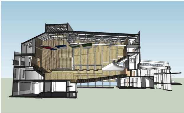
君山音樂廳剖面圖
