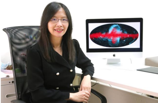
本校天文所楊湘怡助理教授以電腦模擬證實銀河系巨大 泡泡為黑洞能量噴發形成。
