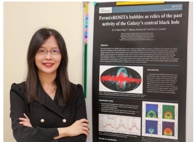
本校天文所楊湘怡助理教授揭開銀河系巨大泡泡成因之 謎。
