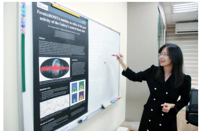
楊湘怡老師解釋，黑洞能量噴發會形成上下對稱的兩個巨 大蕈狀泡泡。
