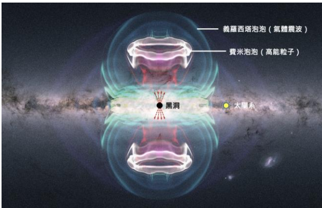
260 萬年前黑洞能量噴發，形成費米泡泡（紅色內圈）與 義羅西塔泡泡（綠色外圈）。
