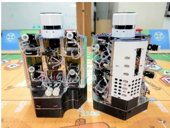
清華機器人此次出賽加裝了多感測器定位系統與全向式底盤，成為致勝關鍵。
