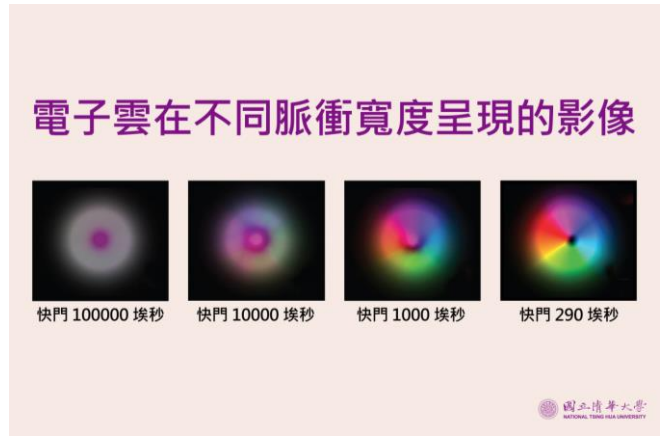
電子雲在不同脈衝寬度呈現的影像
