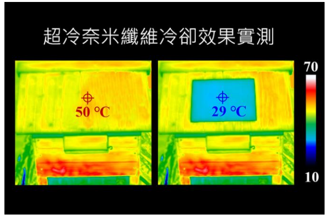
將超冷奈米纖維鋪在模型屋屋頂，經紅外光熱像儀測量，溫度從攝氏 50 度降到 29 度。
